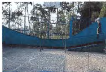
Fotografía 8 MANTENIMIENTO DE BARANDA DE METAL
